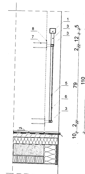
PRZEKRÓJ I-I
